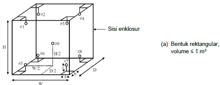
Gambar penempatan sensor
